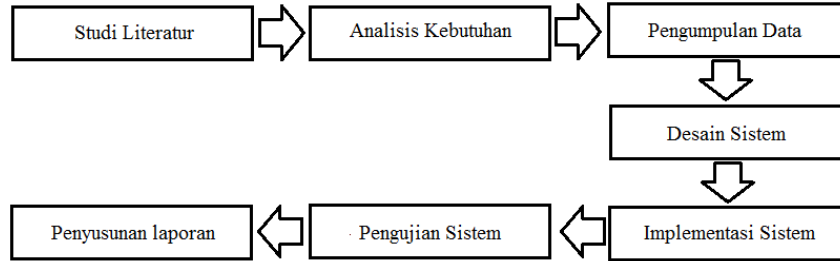
Gambar 1. Alur Analisis
